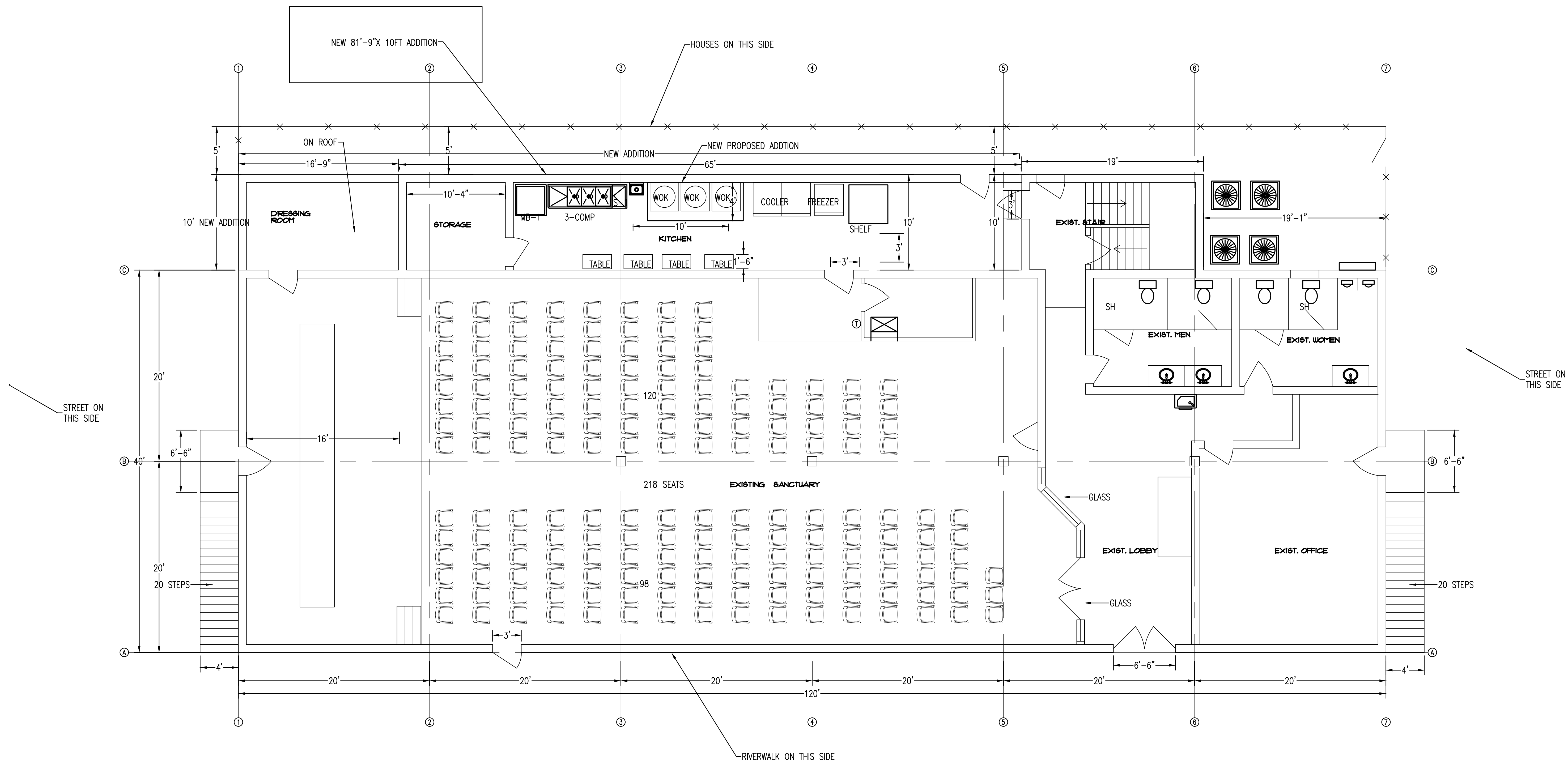
1 FLOOR PLAN A-3 SCALE: 3/16" = 1' - 0"
